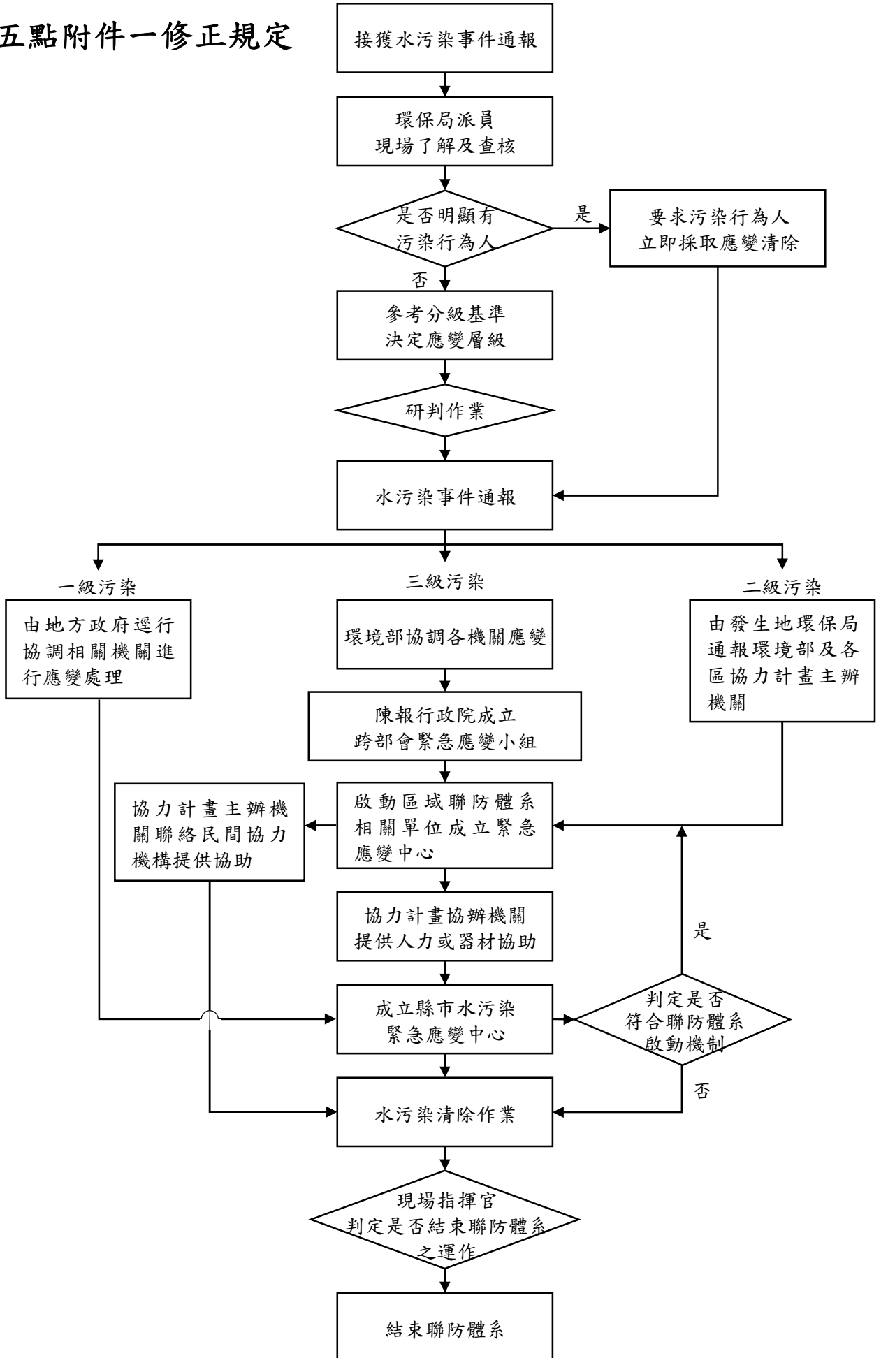
附件一、水污染事件應變作業流程圖
