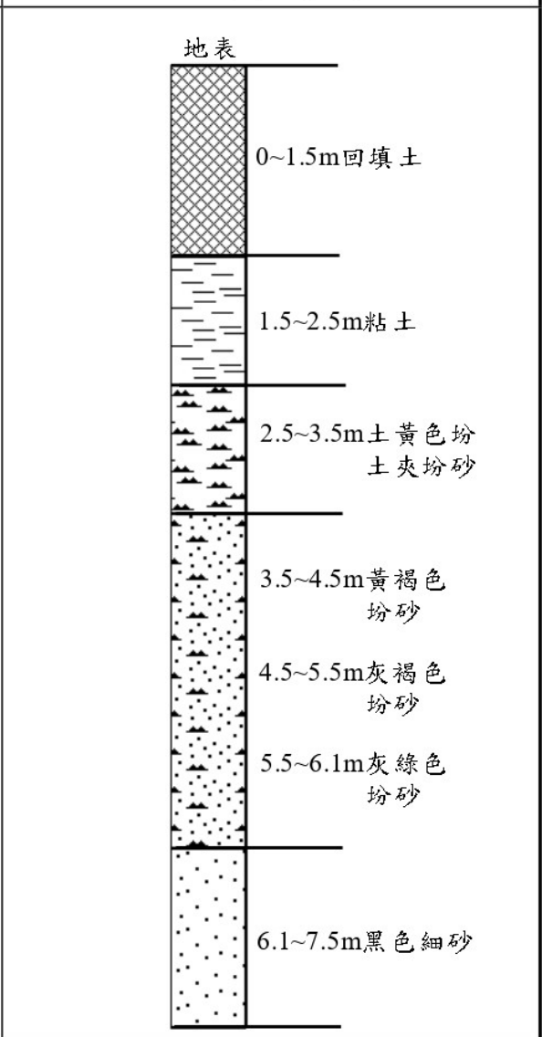
地質剖面圖
