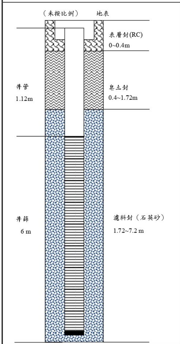
監測井構造圖
